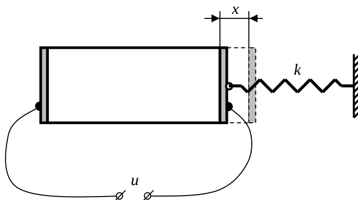
Рис. 1. Пьезоэлектрический преобразователь с упругой нагрузкой
