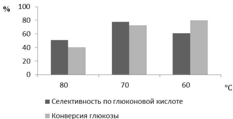
Рис. 2. Сравнительная диаграмма селективности и конверсии при разных температурных условиях
