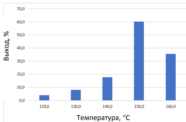
Рис. 4. Зависимость выхода ксилозы от температуры реакции ( \tau = 1 ч)
