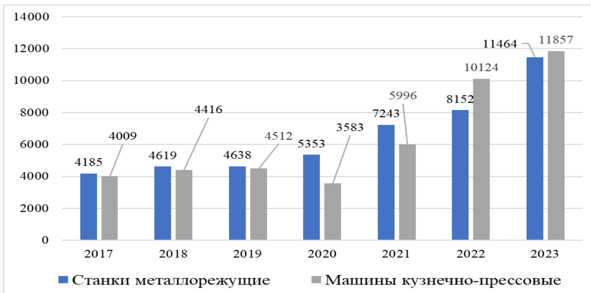
Рис. 4. Объем производства станков, ед. оборуд., в период с 2017 по 2023 годы (составлено авторами по данным [6])
