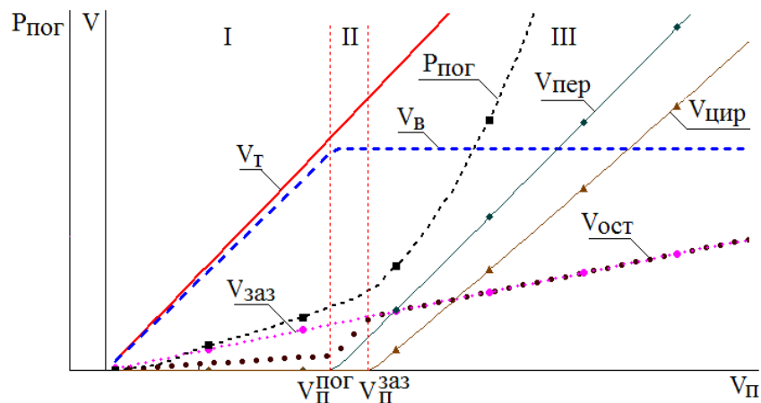
Рис. 3. Графическое представление процесса погрузки: V_{\text{Пог}}^{\text{П}} и V_{\text{П}}^{\text{заз}} – скорости перемещения, соответствующие границам первого и второго диапазона соответственно
