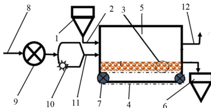
Рис. 1. Технологическая схема сушилки какао-бобов: 1 – вход; 2 – входной поток; 3 – слой какао-бобов; 4 – конвейерная лента; 5 – сушильная камера; 6 – выходной поток; 7 – мотор конвейера; 8 – сушильный воздух на впуске; 9 – вентилятор; 10 – нагреватель; 11 – поток горячего воздуха; 12 – выходной поток воздуха
