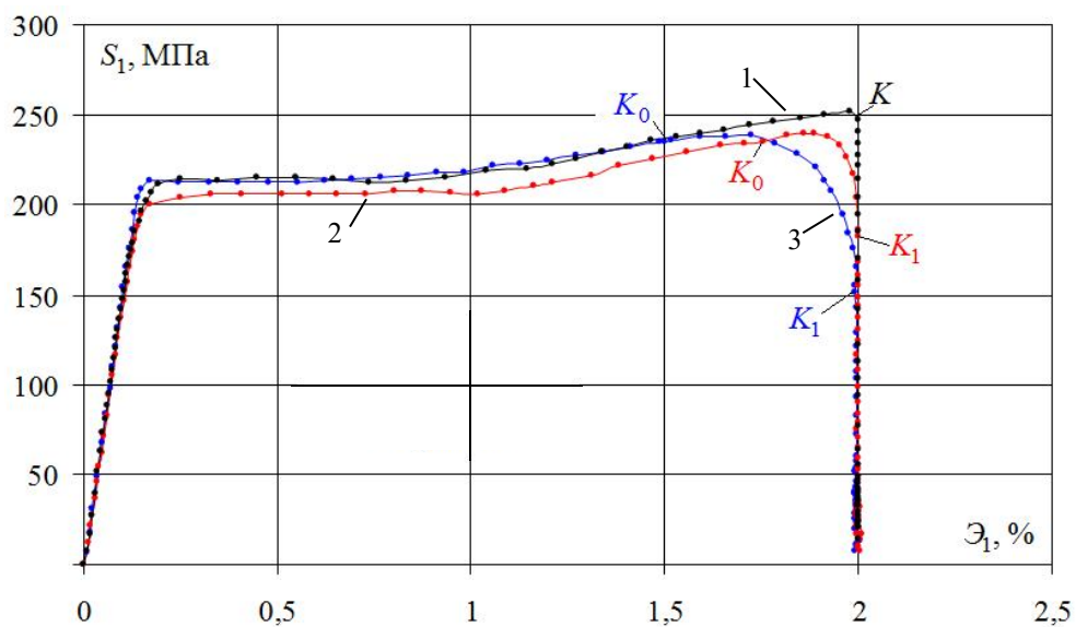
Рис. 5. Локальная диаграмма деформирования S_1 - \varepsilon_1 : 1-3 – образцы
