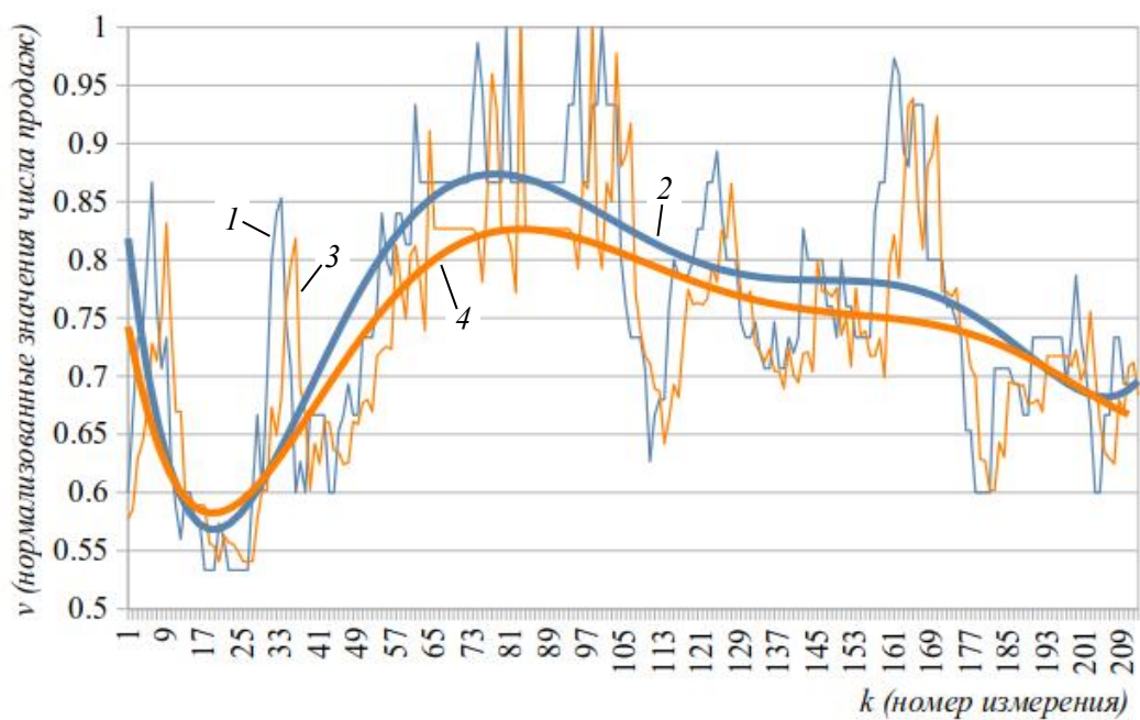
Рис. 3. Соответствие предсказанных и действительных значений ДП: а – обучающий набор, нормализованные значения; б – проверочный набор, нормализованные значения: 1, 3 – действительные значения; 2 – линия тренда для действительных значений (полиномиальная регрессия); 4 – линия тренда для предсказанных значений (полиномиальная регрессия)
