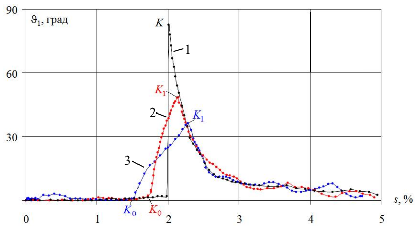
Рис. 4. Диаграмма характеристики векторных свойств материала: 1-3 – образцы
