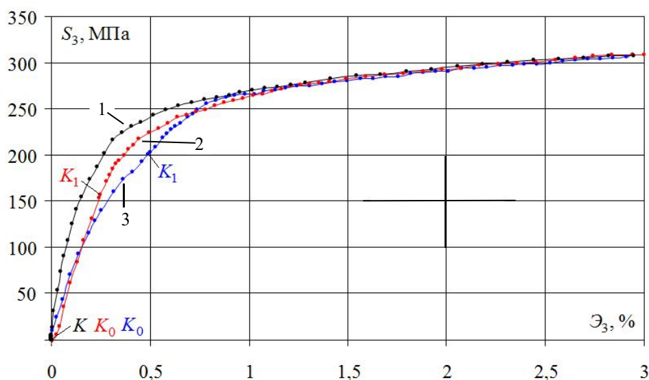
Рис. 6. Локальная диаграмма деформирования S_3 – \varepsilon_3 : 1–3 – образцы
