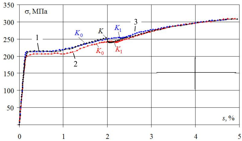
Рис. 3. Диаграмма деформирования \sigma - s : 1-3 – образцы
