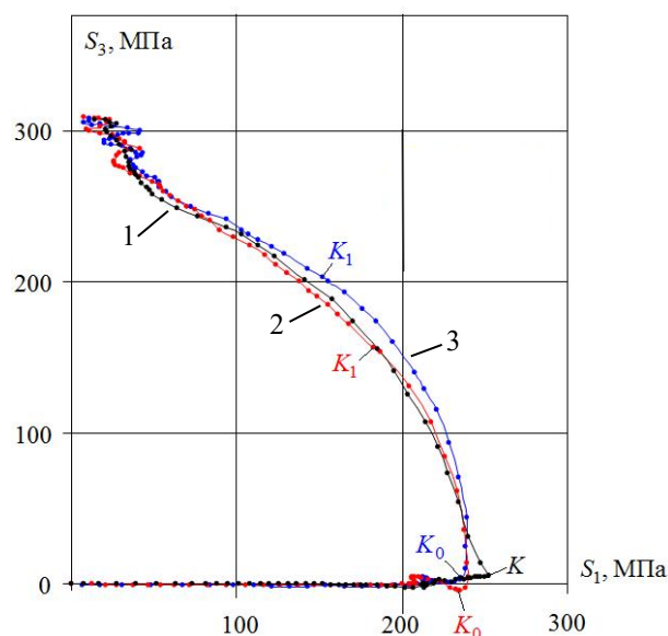
Рис. 2. Отклик по напряжениям на плоскости S_1 – S_3 : 1–3 – образцы
