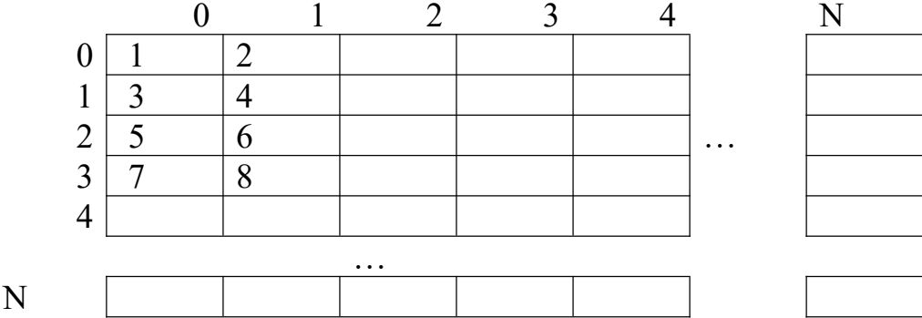
Рис. 3. Пример GPU-сетки с массивом
