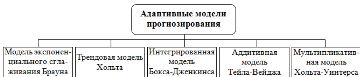
Рис. 1. Основные виды адаптивных моделей прогнозирования
